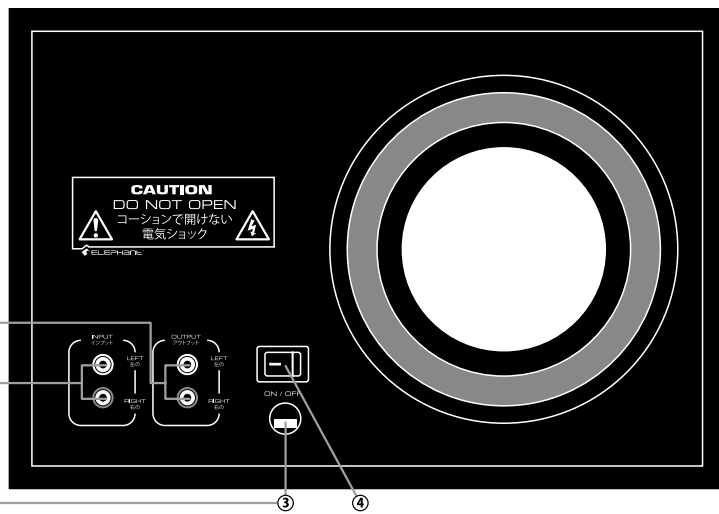
Subwoofer (front view) サブウーファー (正面図)
